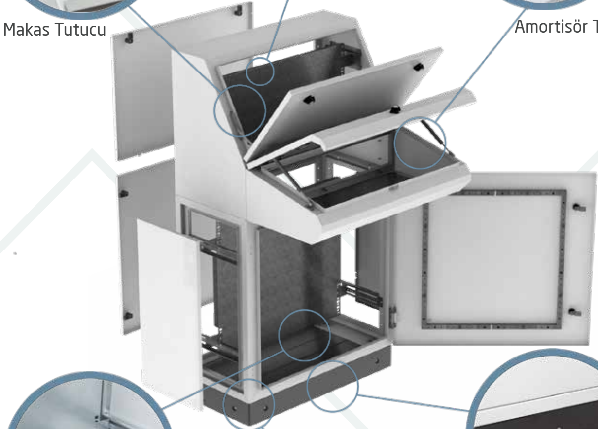
Açı Ayarlı Montaj Plakası
